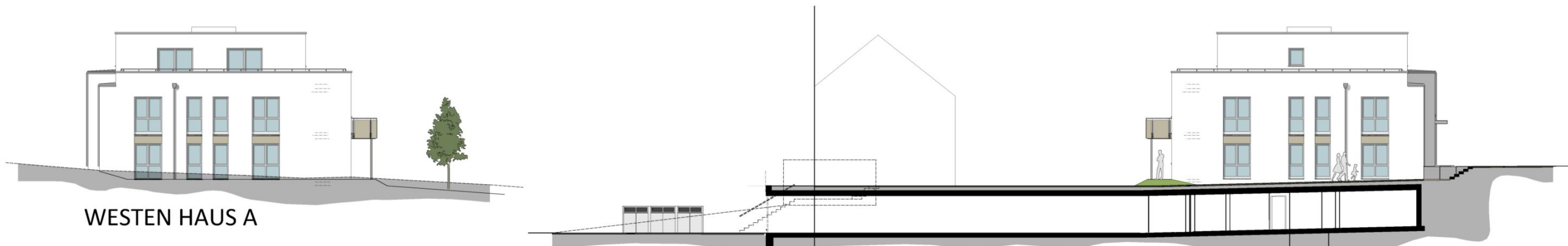
SCHNITT 3-3
